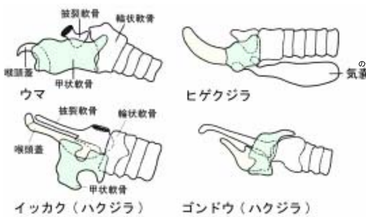
図 陸上哺乳類と海生哺乳類の喉頭の構造 Hearing by Whales and Dolphins P.453 Fig.10.19 より改変
