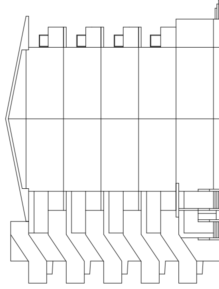
南棟 南西側立面図
