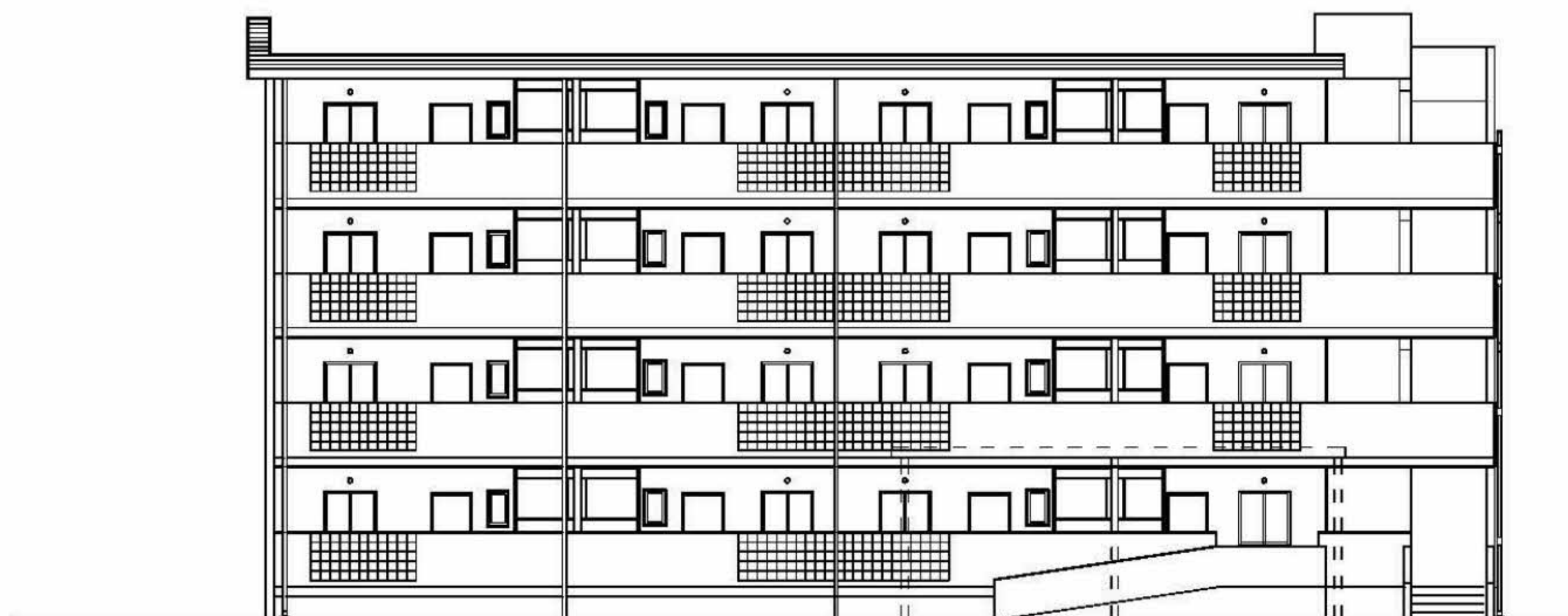
北側立面図
