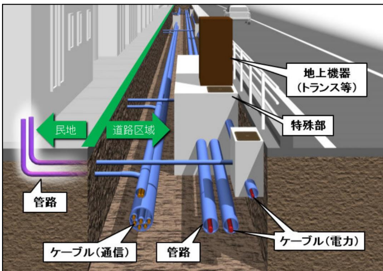
電線共同溝イメージ
