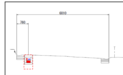
整備イメージ及び計画道路断面図
